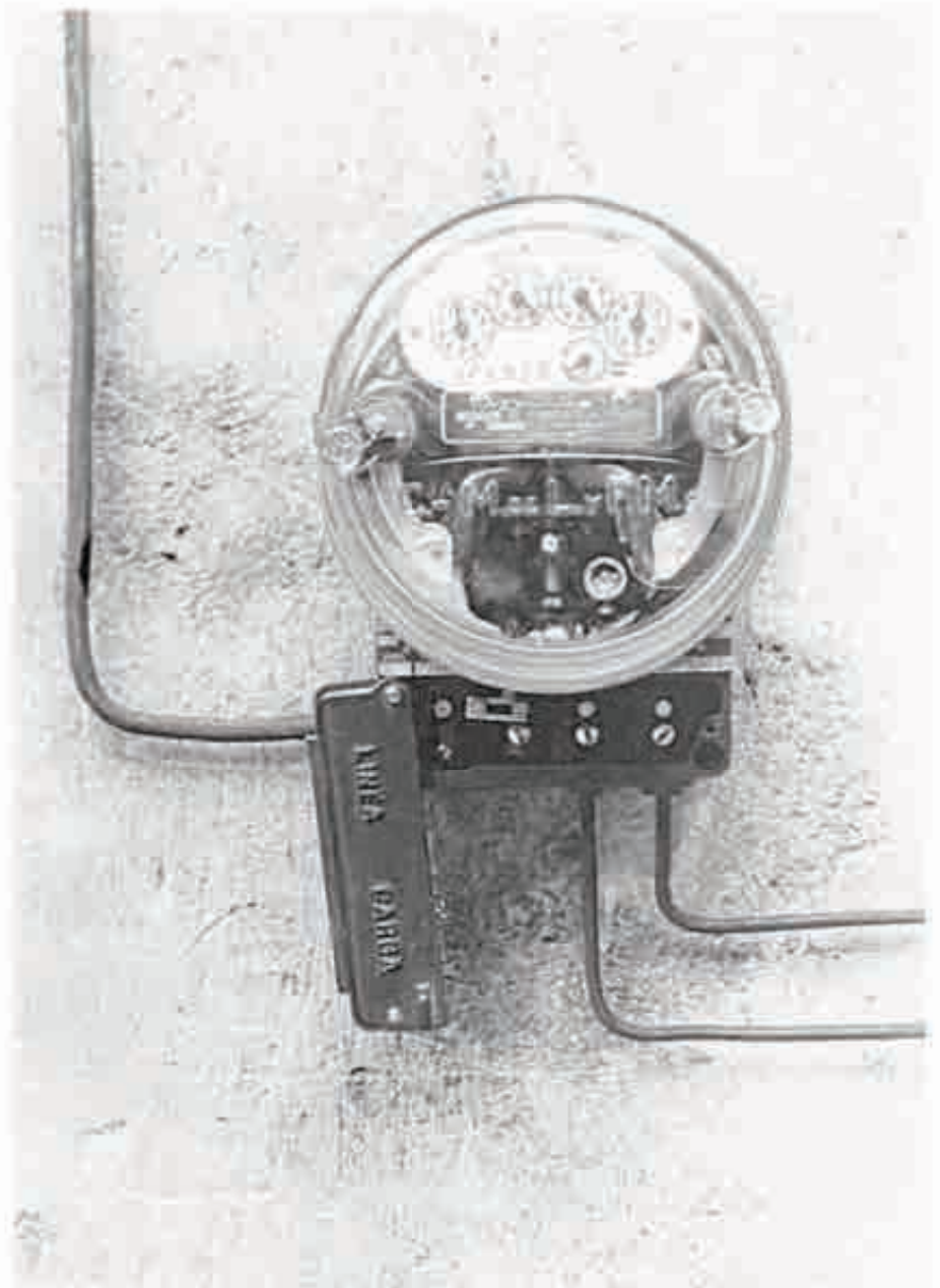
Medidor doméstico instalado por la Mexican Light & Power Company Limited, 1922. Fototeca de Luz y Fuerza del Centro. Archivo Histórico.
