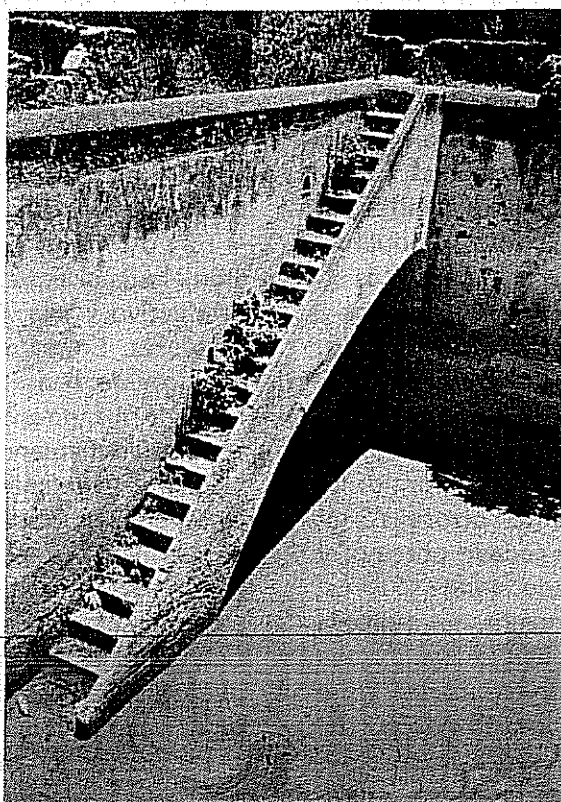
Cisterna o aljibe. Santa Bárbara, municipio de Huamantla
