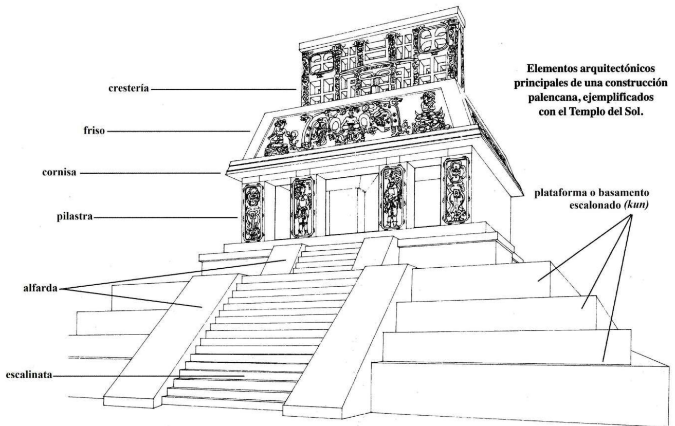
Figura 7. Elementos arquitectónicos típicos de los edificios del Grupo de las Cruces ejemplificados con el Templo del Sol. Dibujo de G. F. Andrews y J. E. Thompson.
